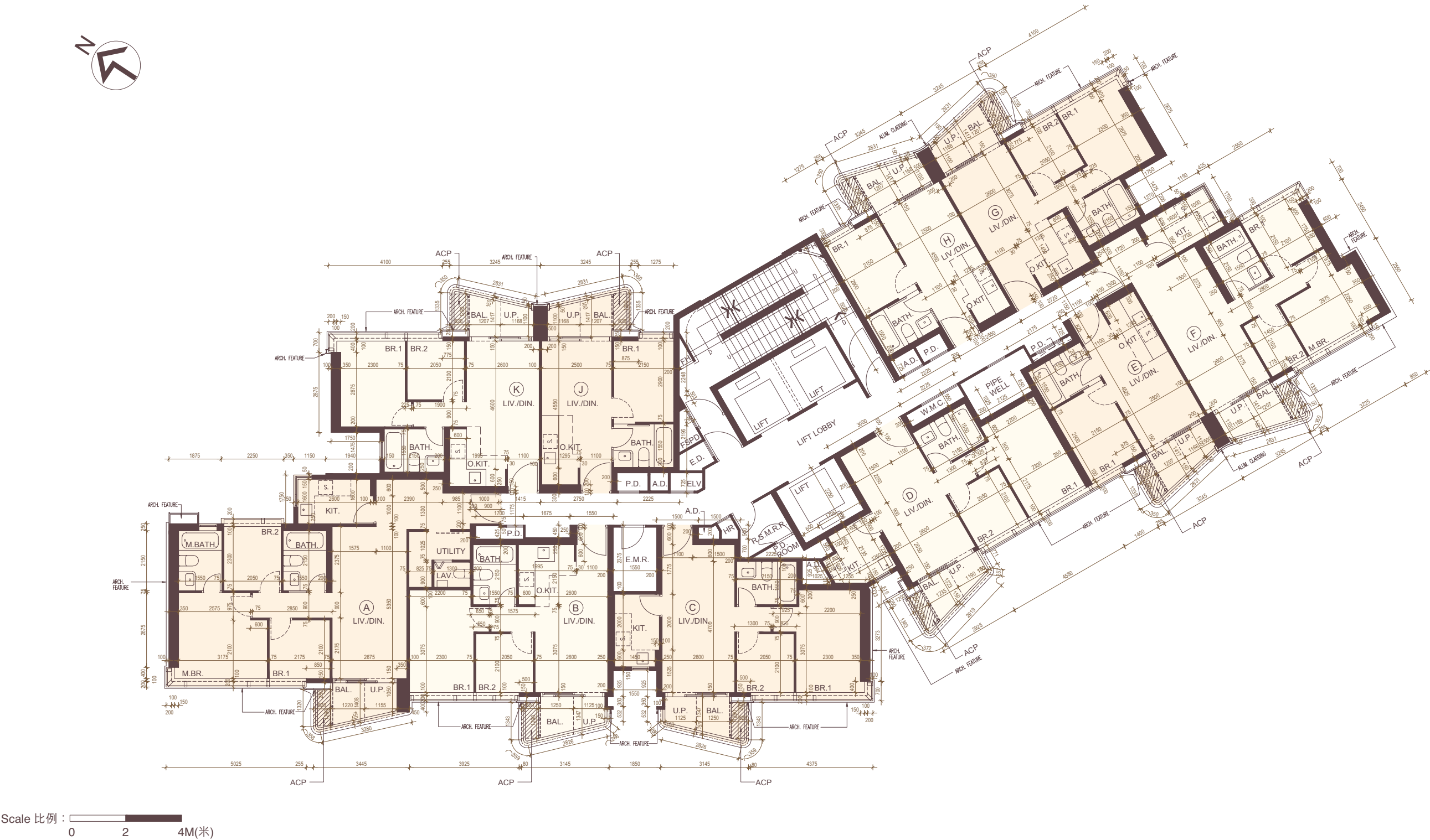
21/F - 23/F, 25/F - 33/F and 35/F - 36/F FLOOR PLAN 21樓至23樓、25樓至33樓及35樓至36樓平面圖
